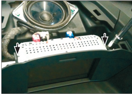
8. Unclip display
