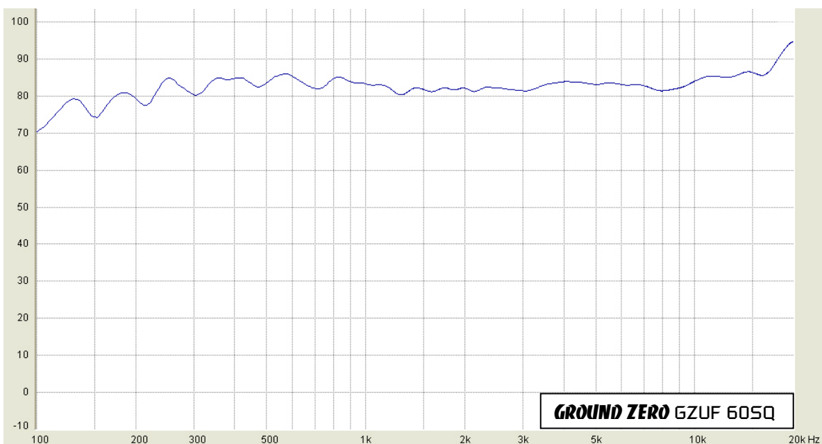
FREQUENZGANG AUF ACHSE / FREQUENCY RESPONSE ON AXIS
