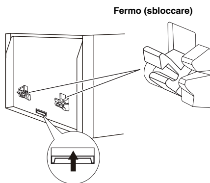
Leva di sblocco
