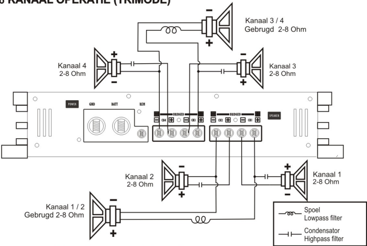
Waardes voor 6dB Passief filtering
