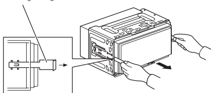
Entriegelungsschlüssel
