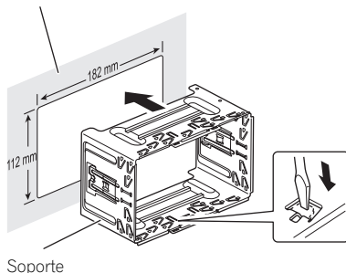
Soporte
