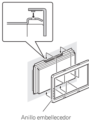
Anillo embellecedor
