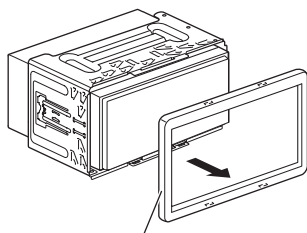
Anillo embellecedor
